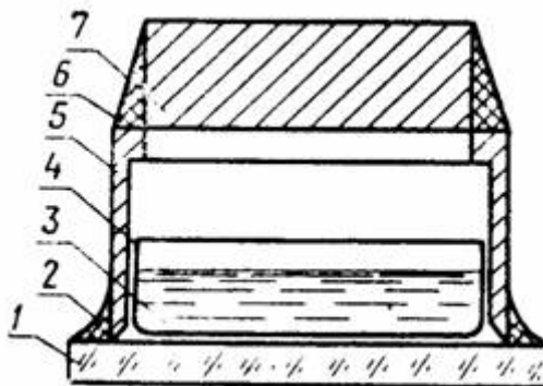
Схема прибора для определения паропроницаемости
